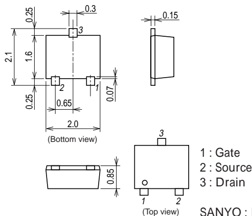
外形図 2167A
